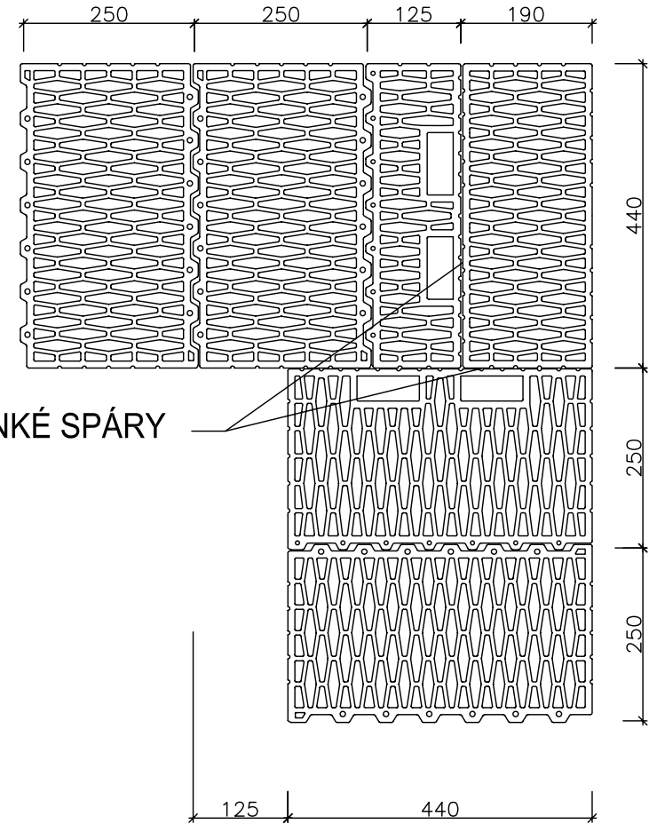
POROTHERM 44 CB VAZBA ROHU
